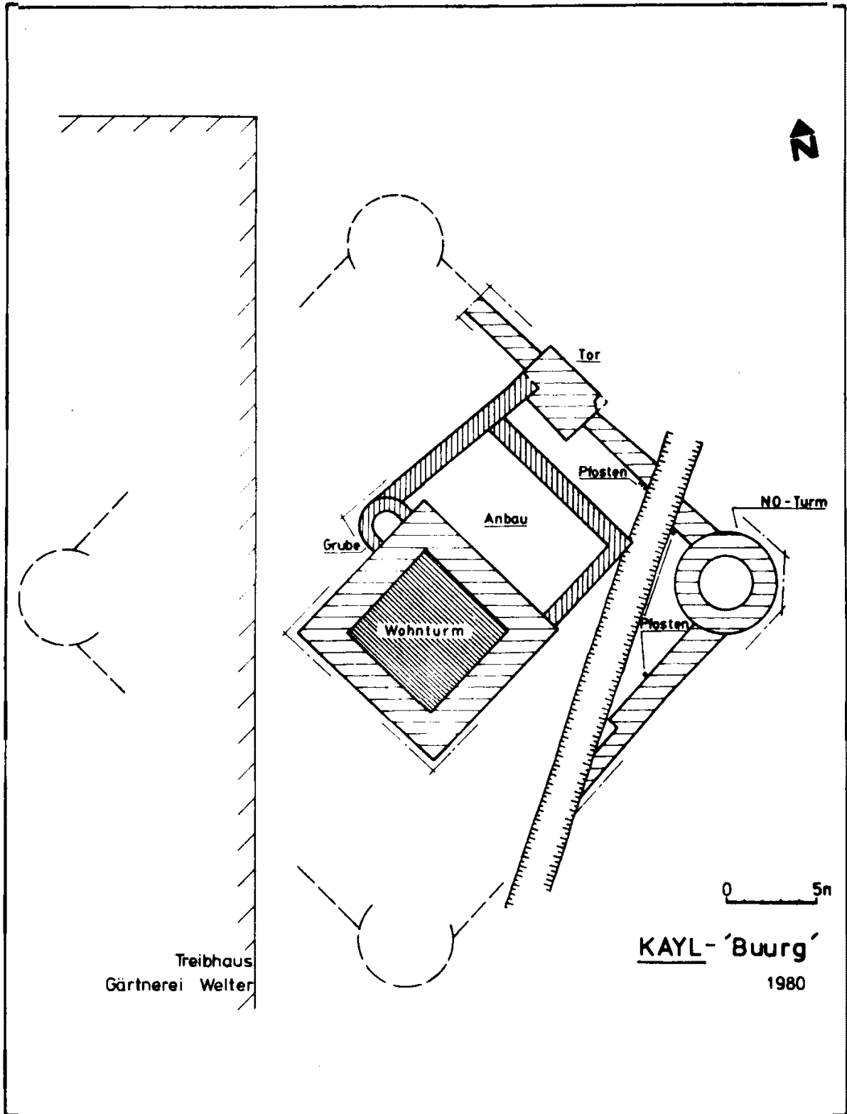
Abb. 2 - Grundriss der Kayler Wasserburg (Zeichnung R. Bis)
