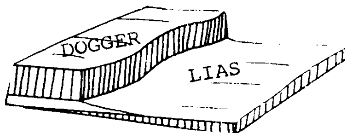
I. Schema der beiden Gesteinsformationen nach dem Entstehen der Doggerformation.
